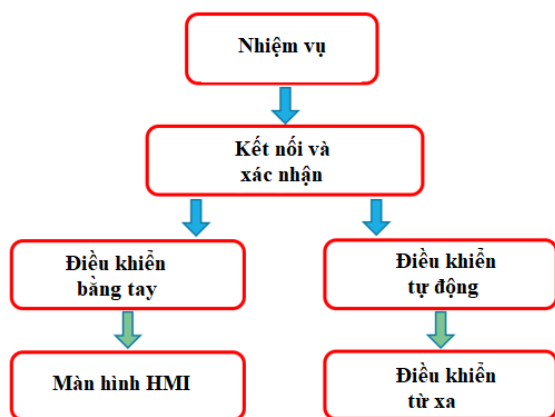
Hình 8. Quy trình và các trạng thái vận hành G2J.
